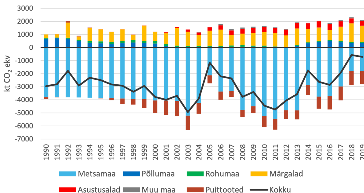
Joonis 23. Kasvuhoonegaaside heide ja sidumine Eesti LULUCFi sektoris 1990–2019
